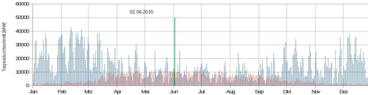
Diagramm 7: Windstromerzeugung und Vergleich mit Solar (Quelle: Windjournal)
