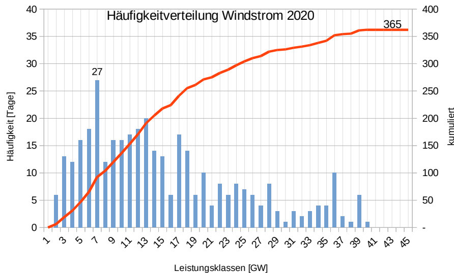
Diagramm 8: Histogramm Windstromerzeugung (Quelle: B. Zierenberg)
