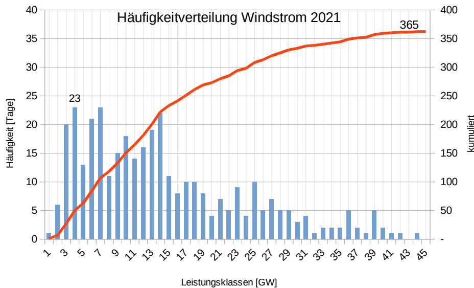
Histogramm Windstromeinspeisung (Quelle: B. Zierenberg)
