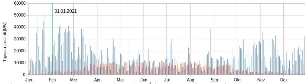
Windstromeinspeisung und Vergleich mit Solar (Quelle: Windjournal)
