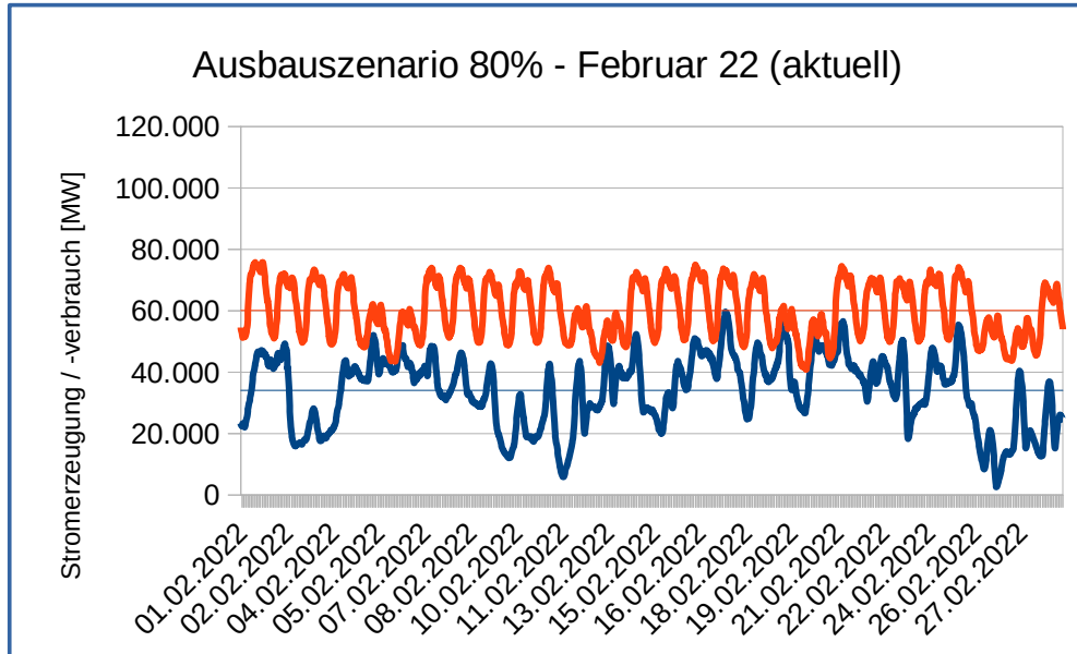
Diagramm 1: Verläufe von Stromerzeugung aus Wind + PV und Stromverbrauch bei aktuellem Ausbaustatus Januar 2022
