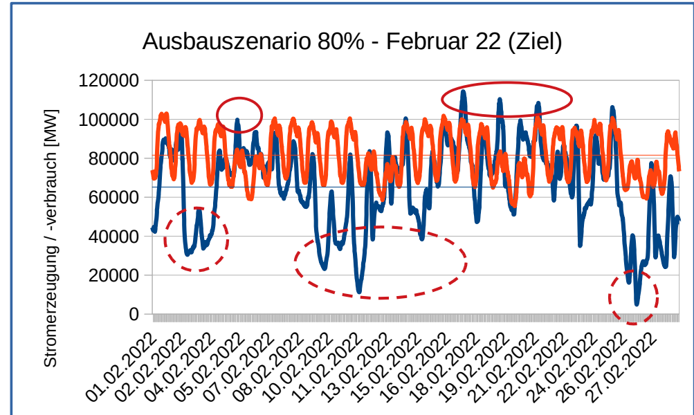
Diagramm 2: Verläufe von Stromerzeugung aus Wind + PV und Stromverbrauch hochgerechnet nach Planungsziel BMWK Februar 2022
