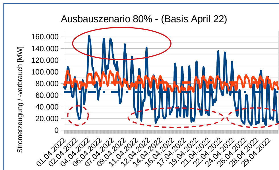
Diagramm 2: Verläufe von Stromerzeugung aus Wind + PV und Stromverbrauch, hochgerechnet aus April 22 entspr. Planungsziel BMWK für April 2030
