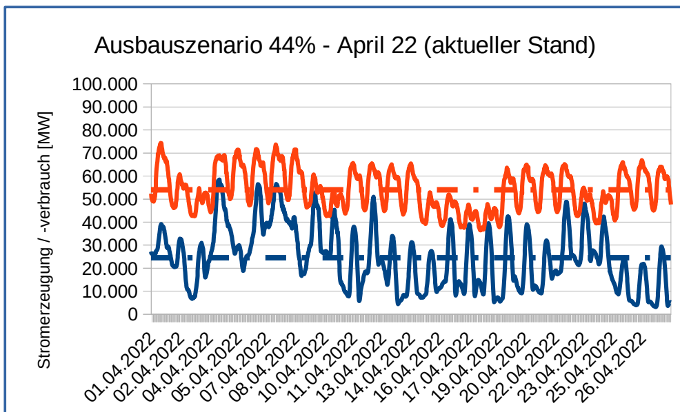
Diagramm 1: Verläufe von Stromerzeugung aus Wind + PV und Stromverbrauch bei aktuellem Ausbaustatus April 2022
