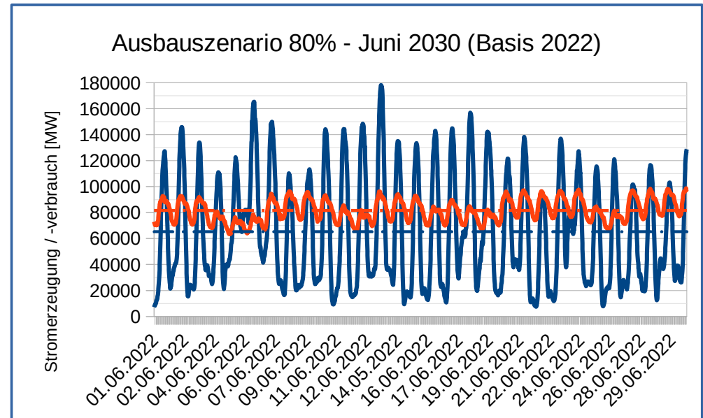
Diagramm 2: Verläufe von Stromerzeugung aus Wind + PV und Stromverbrauch, hochgerechnet aus Juni 22 entspr. Planungsziel BMWK für Juni 2030
