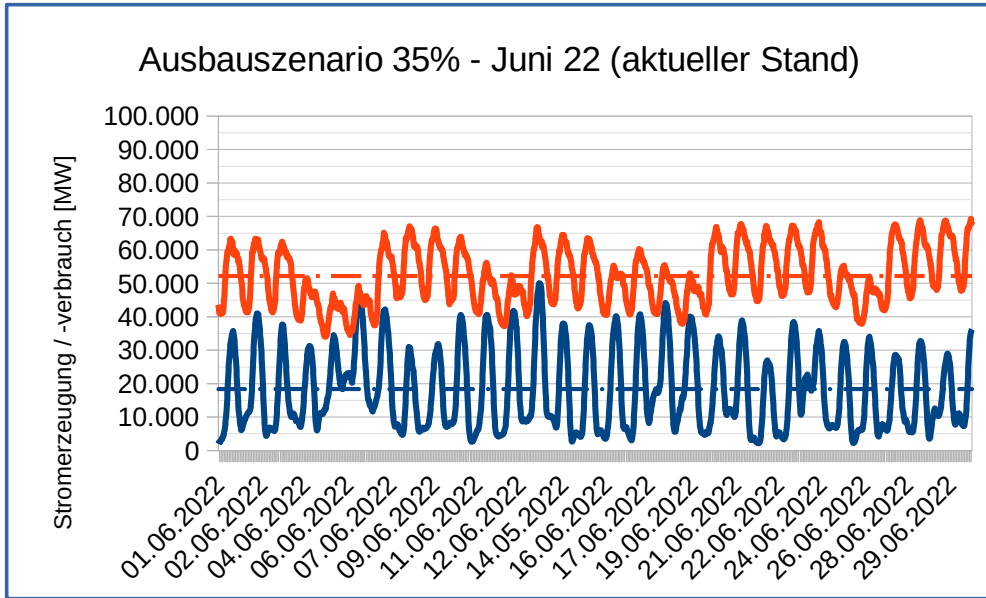
Diagramm 1: Verläufe von Stromerzeugung aus Wind + PV und Stromverbrauch bei aktuellem Ausbaustatus Juni 2022
