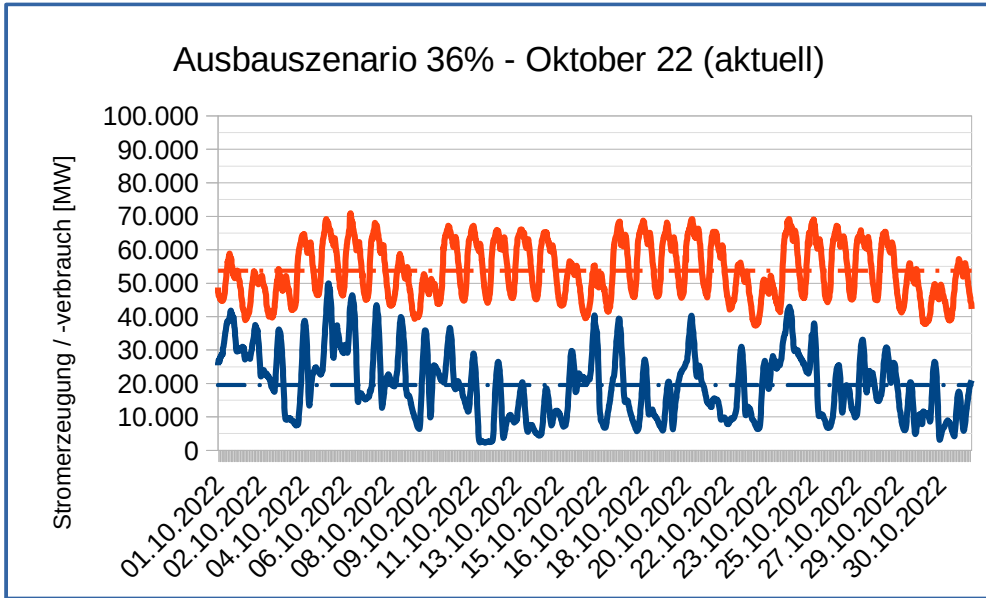
Diagramm 1: Verläufe von Stromerzeugung aus Wind + PV und Stromverbrauch bei aktuellem Ausbaustatus Oktober 2022
