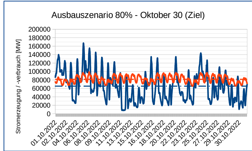
Diagramm 2: Verläufe von Stromerzeugung aus Wind + PV und Stromverbrauch, hochgerechnet aus Oktober 22 entspr. Planungsziel BMWK für Oktober 2030
