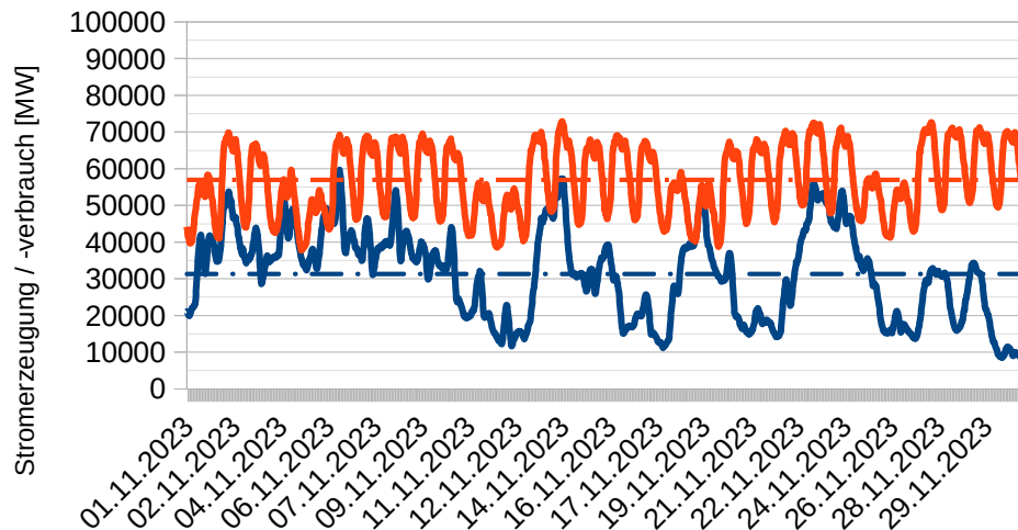
Diagramm 1: Verläufe von Stromerzeugung aus Wind + PV und Stromverbrauch bei aktuellem Ausbaustatus November 2023
