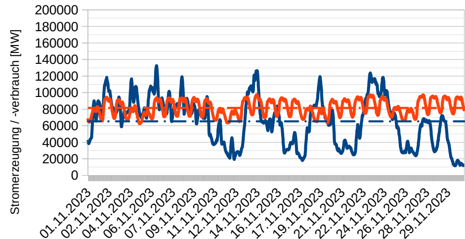
Diagramm 2: Verläufe von Ökostromerzeugung (Wind, PV, Biomasse und Wasserkraft), hochgerechnet aus November 2023 entspr. Planungsziel BMWK für November 2030
